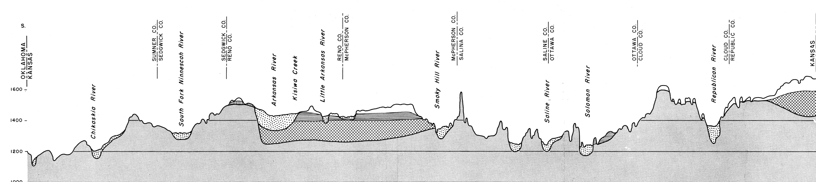
C—C'
